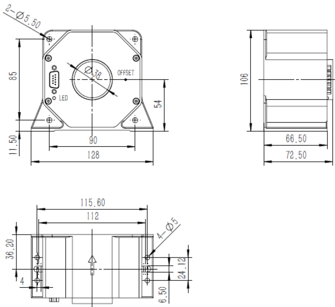
图 1 外形图
