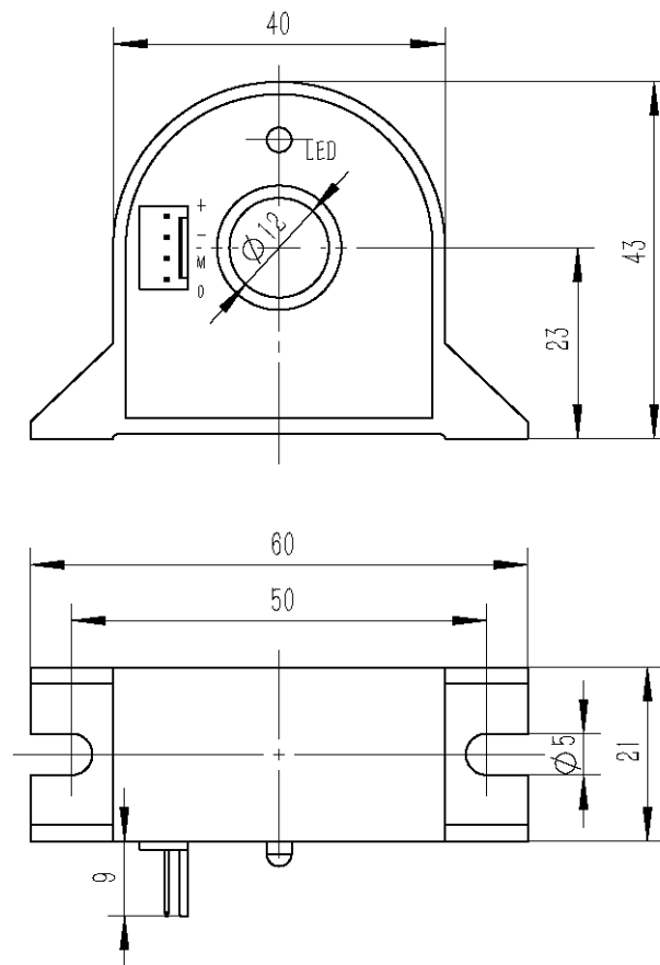
图 1 外形图
