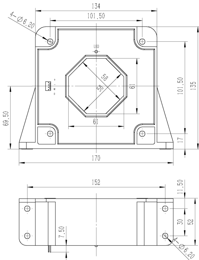
图 1 外形图
