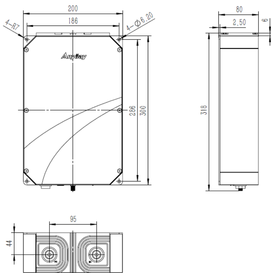
图 1 外形尺寸图
